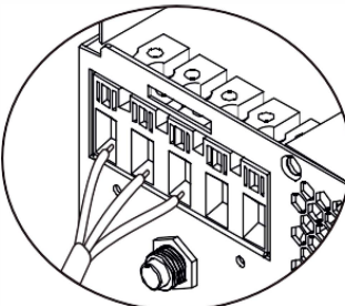
1 kW @-> földelés (sárgászöld) / L-> vezeték (barna vagy fekete) / N-> semleges (kék) 2-3 kW
